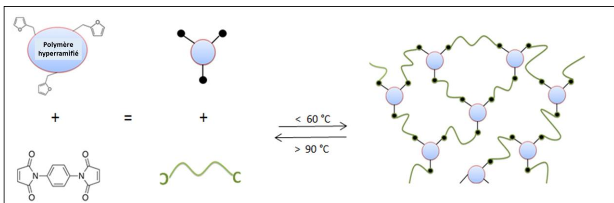
Figure 1 : Exemple d'élaboration d'un réseau macromoléculaire tridimensionnel réversible
